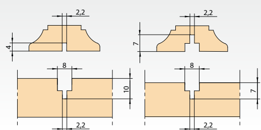
Fräßvariante 1
