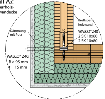
Detail C: Brettsperrholz- Außen- Innenwand- Anschluss
