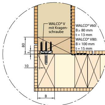
Detail A 2 : Außenwandecke mit Dampfsperre (PE-Folie)
