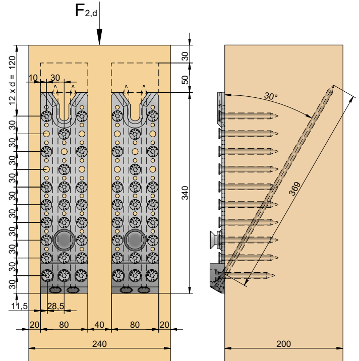
ST. Verschraubung in Stütze
