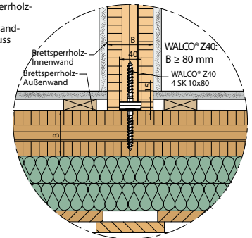
Detail E: Gehrungsanschluss Brettsperrholzwand
