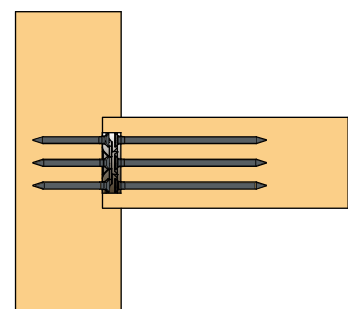
Verbinder untergebracht in Pfette Ende
