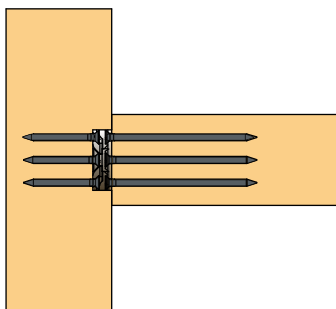
Verbinder im Hauptträger eingegrast
