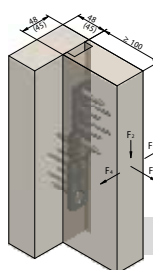
Eckanschluss
