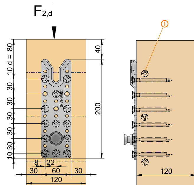
ST. Verschraubung in Stütze
