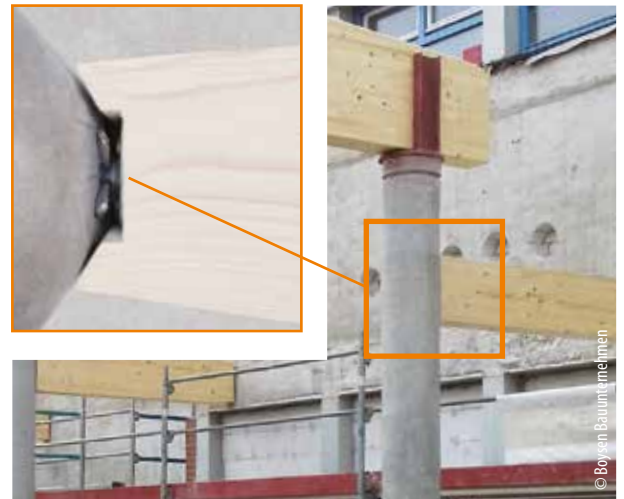
RICON®S Holz-Beton Anschluss
