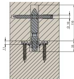
Schnitt A-A
