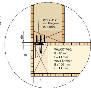
Detail A: Außenwandecke mit durchgehender Holzwerkstoffplatte
