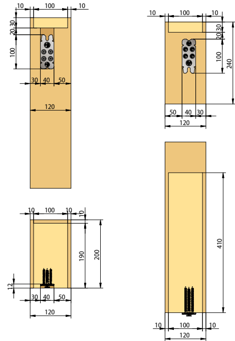
Stützeanschluss
