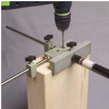
Vorbohren des Nebenträger
