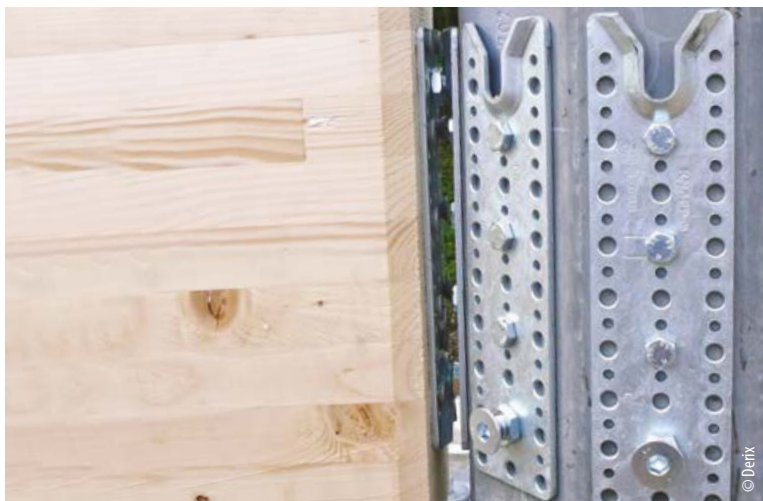
RICON® S 290/80 - jonction acier/bois
