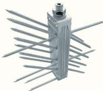
Connecteur MEGANT®
