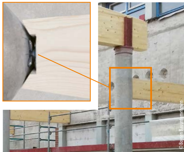
RICON® S - jonction bois/béton
