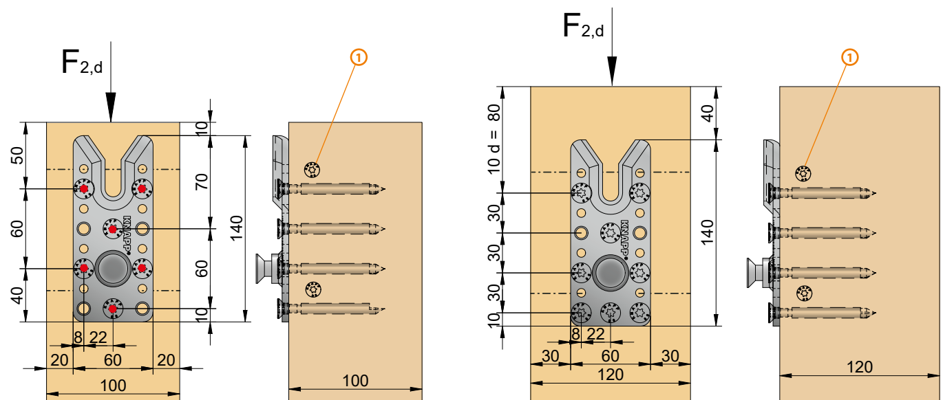
Vissage min. sur poteau
