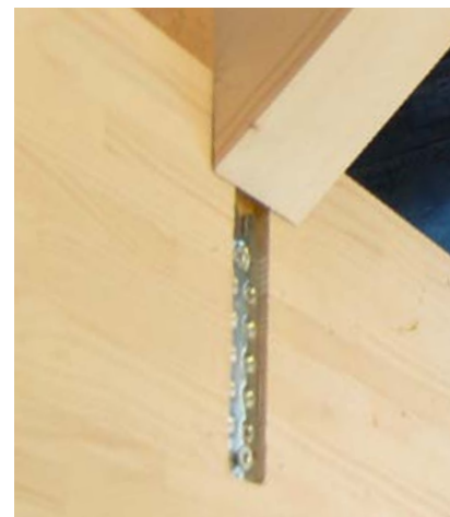
Assemblage de chevron avec RICON® 160/40.
