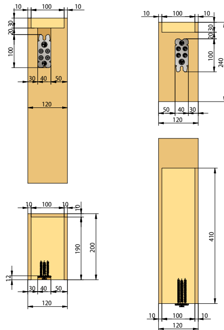
Assemblage sur poteau
