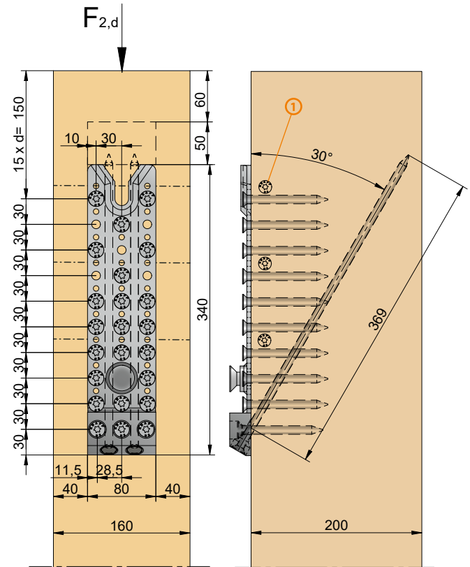
Vissage standard sur poteau
