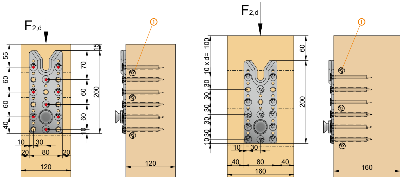
Vissage min. sur poteau
