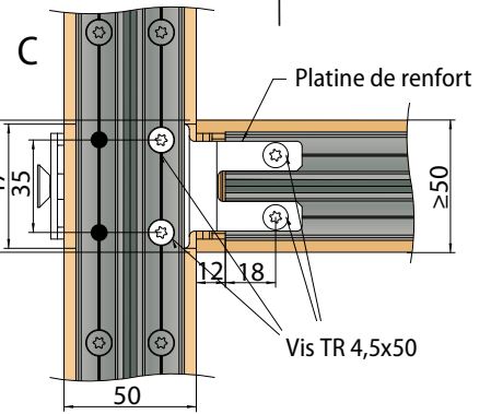
Assemblage double RICON® avec platine de renfort (VP)
