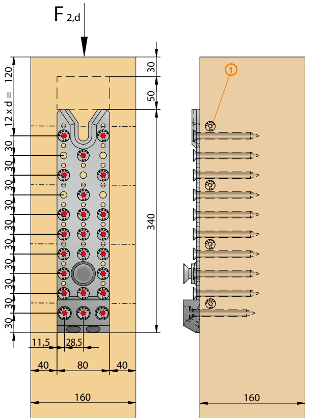
Vissage min. sur poteau
